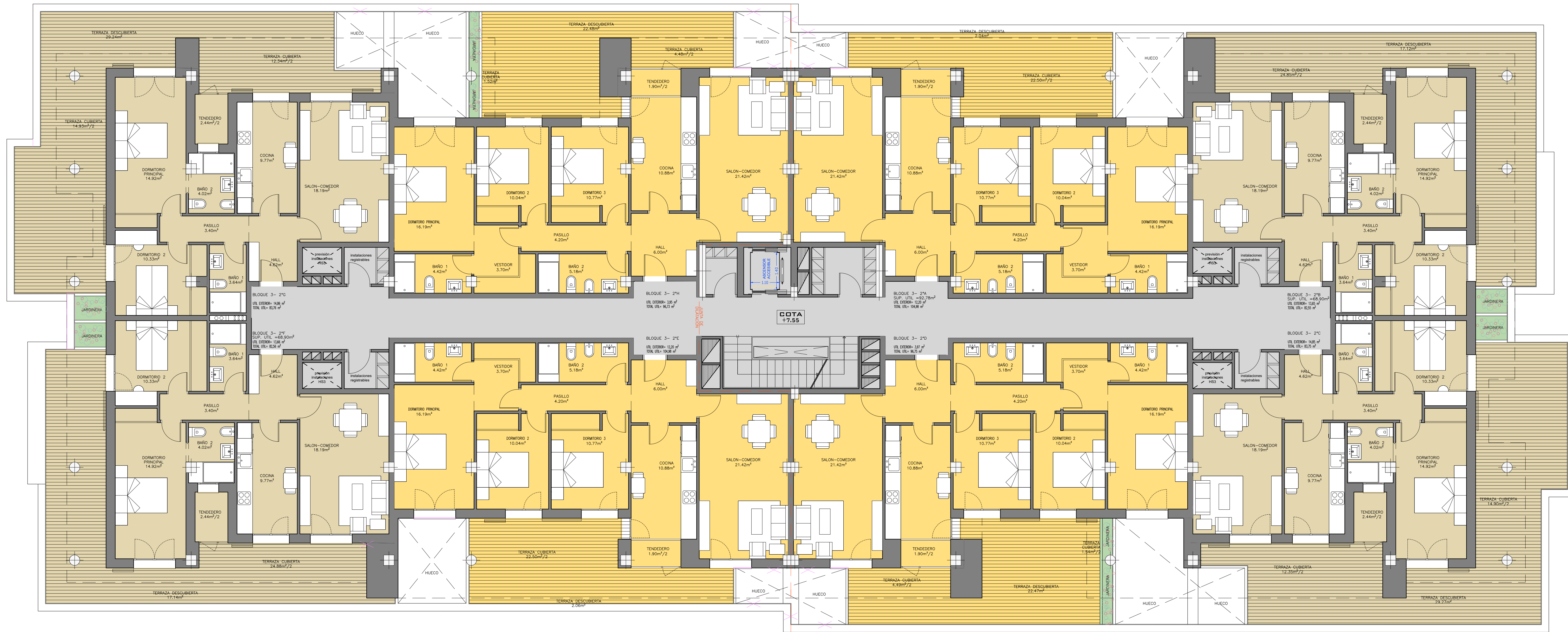
PLANTA SEGUNDA BLOQUE B3
