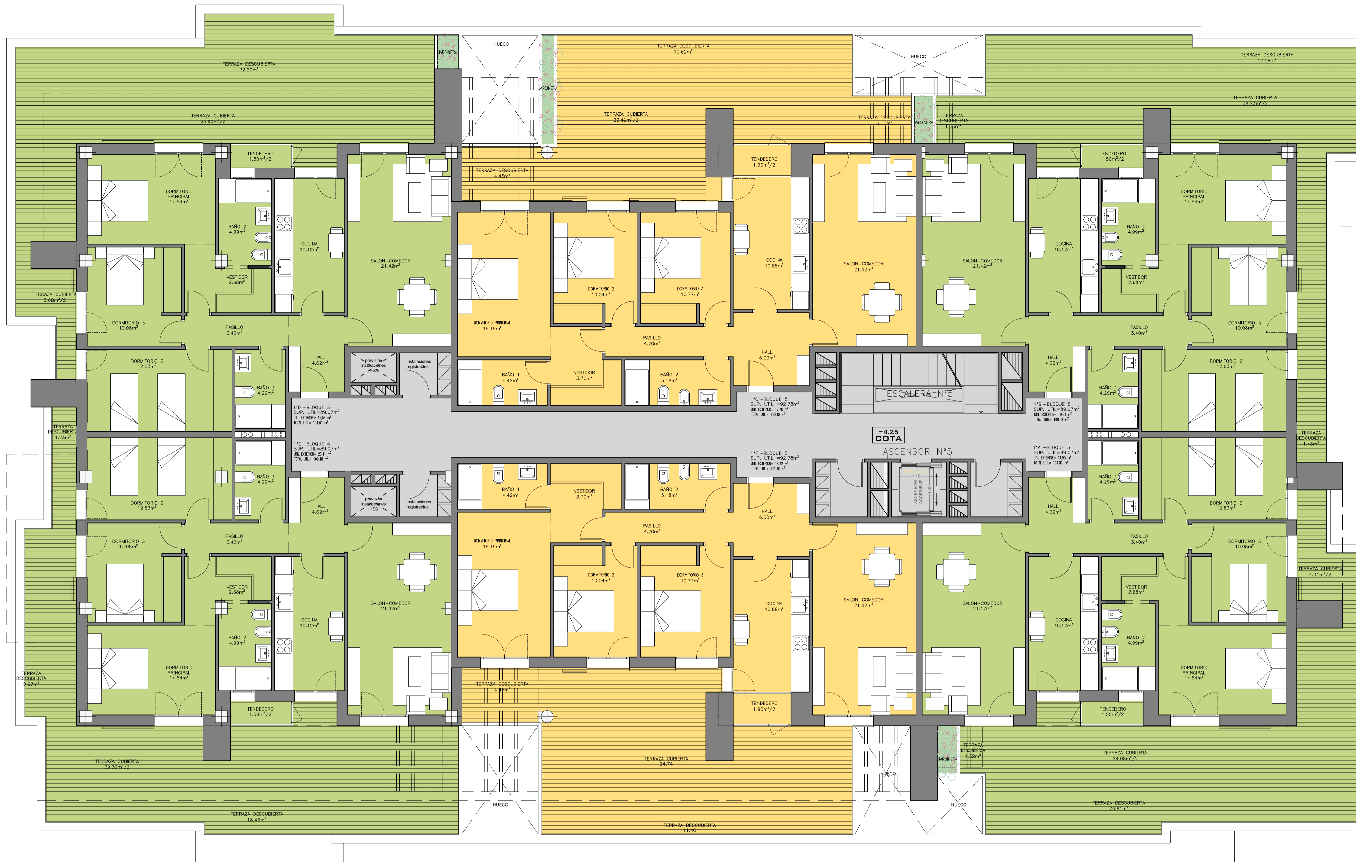
PLANTA PRIMERA BLOQUE B5
